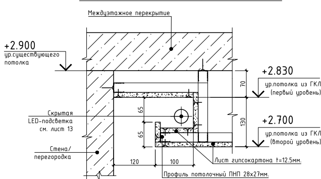
Узел 2 Устройство полки для скрытой подсветки
