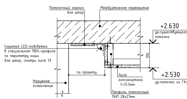
Узел 3 Устройство ниш для скрытого потолочного карниза для штор
