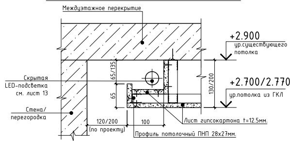
Узел 2 Устройство полки для скрытой подсветки
